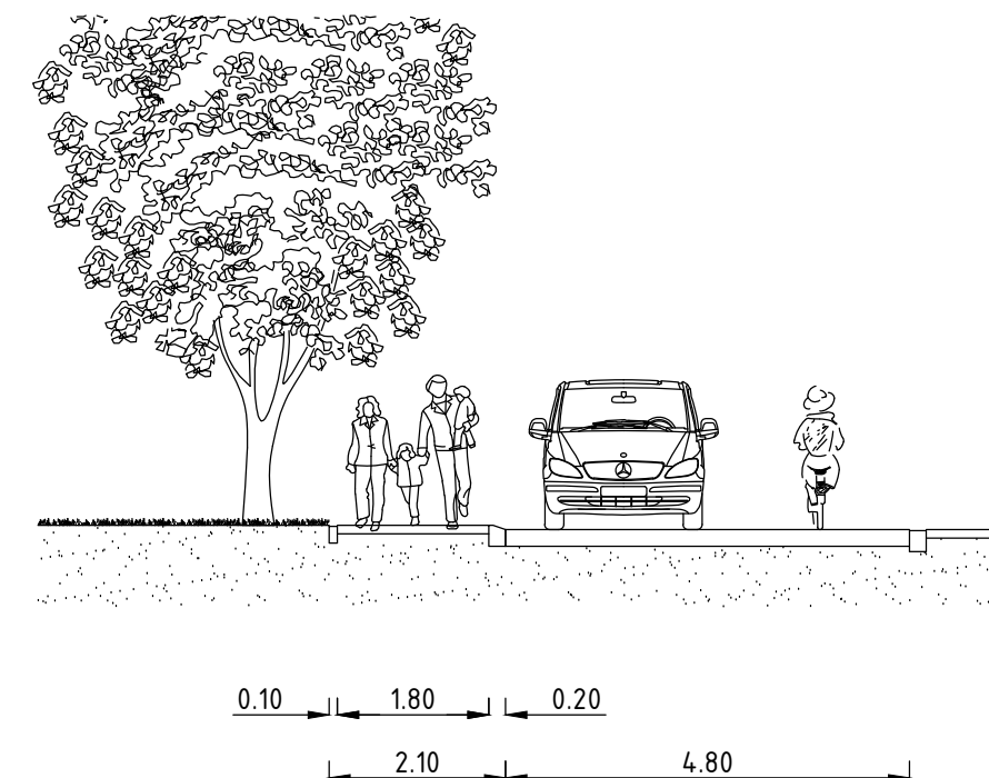
Dwarsdoorsnede B SCHAAL 1:100
