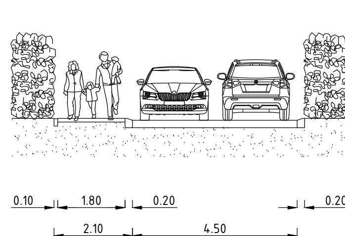
Dwarsdoorsnede C SCHAAL 1:100
