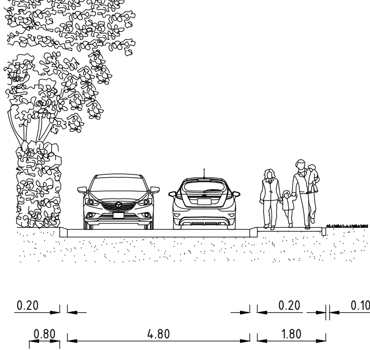
Dwarsdoorsnede A SCHAAL 1:100
