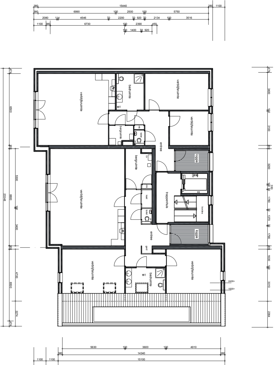
3e verdieping
